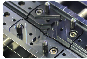
소재 고정용 핀
